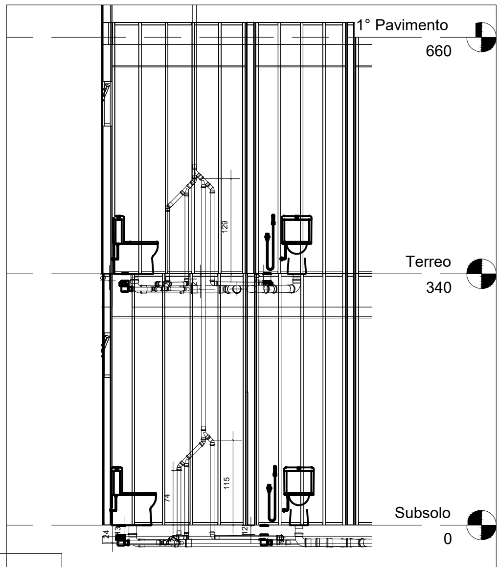
3- Corte 3-ES 1 : 50
