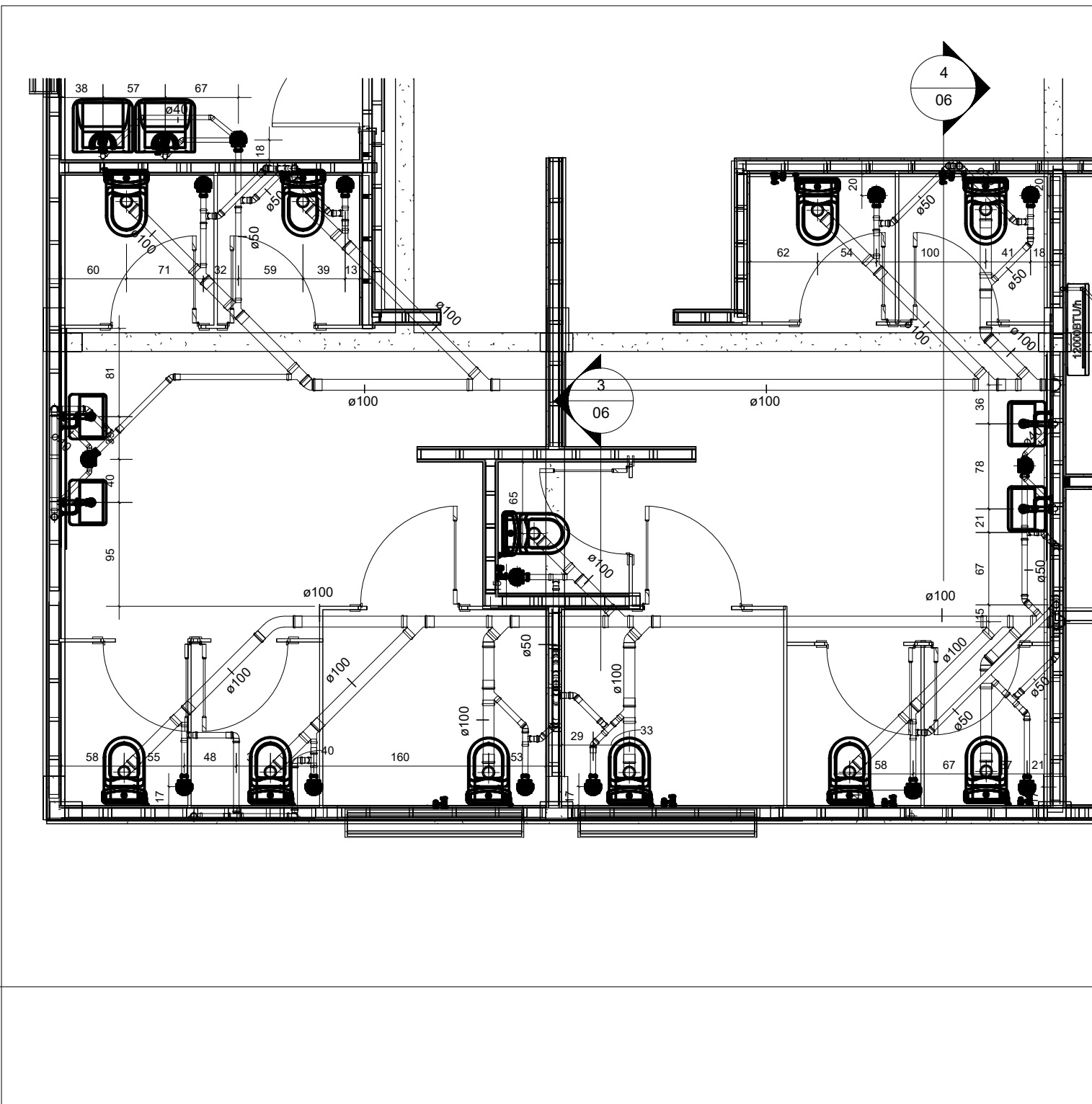
Banheiros 1 : 50
