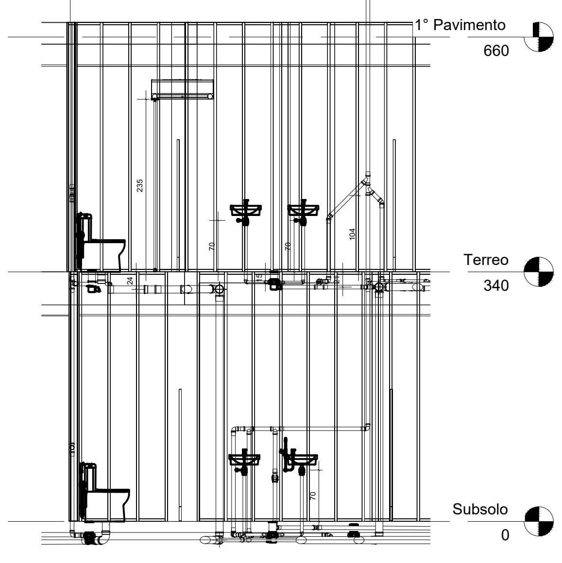
4- Corte 4-ES 1 : 50
